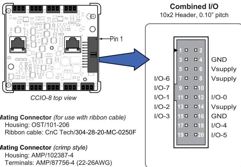
CCIO-8 I/O Header
